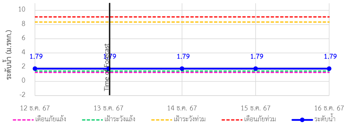
TC220902 สะพานวัดบางดี ต.บางดี อ.ห้วยยอด จ.ตรัง
