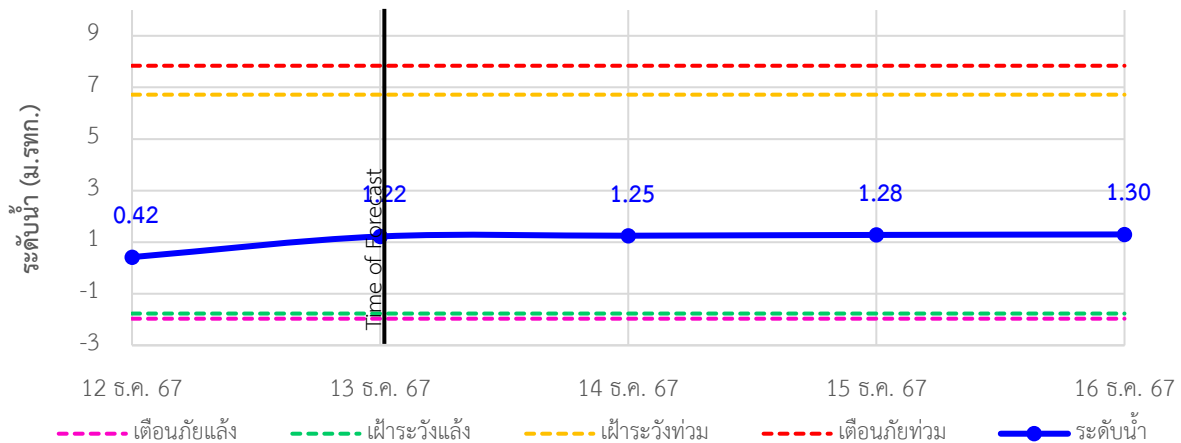
TC220306 สะพานบ้านฝ่ายท่า ตำบลกะเปอร์ อำเภอกะเปอร์ จังหวัดระนอง
